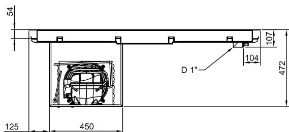
Lato posteriore
